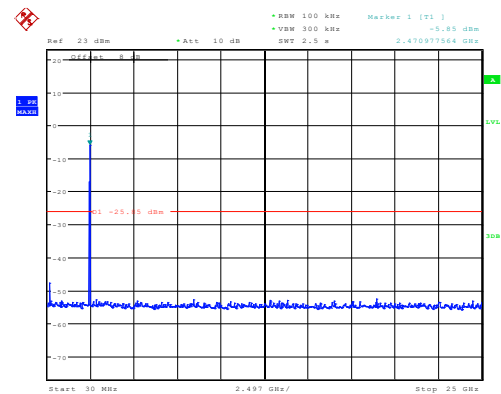
802.11b_2472MHz_Chain 1
