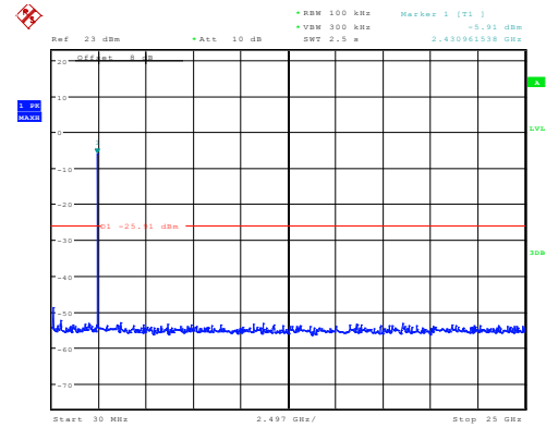
802.11b_2442MHz_Chain 0
