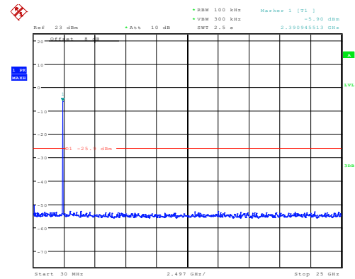
802.11b_2412MHz_Chain 1
