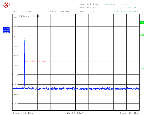
802.11b_2472MHz_Chain 0
