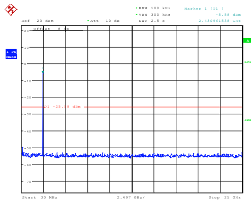
802.11b_2442MHz_Chain 1
