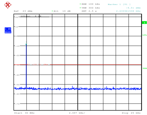
802.11n20_2442MHz_Chain 0
