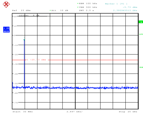
802.11b_2412MHz_Chain 0
