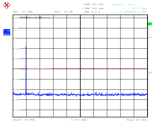
802.11n20_2412MHz_Chain 0
