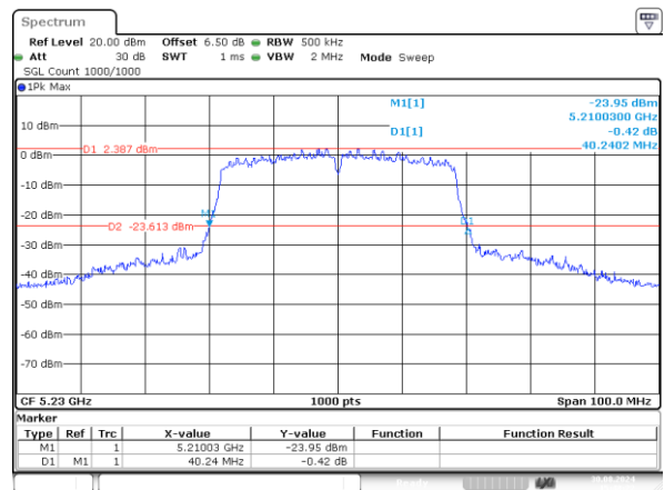
n40_5230MHz_Chain 1 40.240MHz
