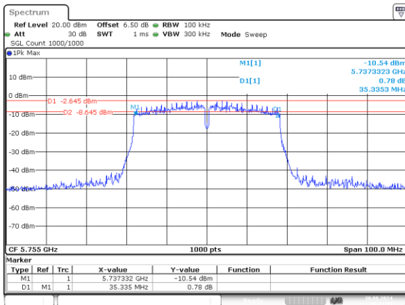
n40_5755MHz_Chain 0 35.335MHz
