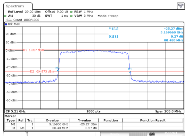
802.11ac80_5210MHz_Chain 1 80.480MHz
