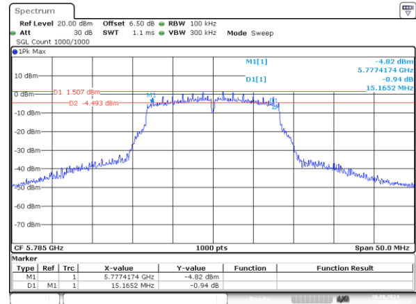
a_5785MHz_Chain 1 15.165MHz
