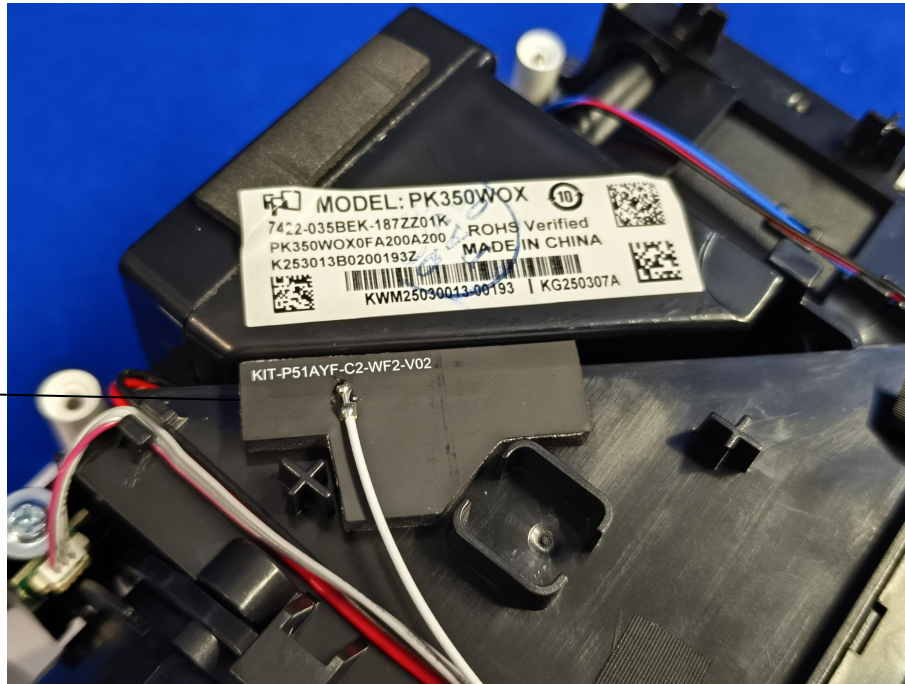
FPC Antenna_WIFI2
