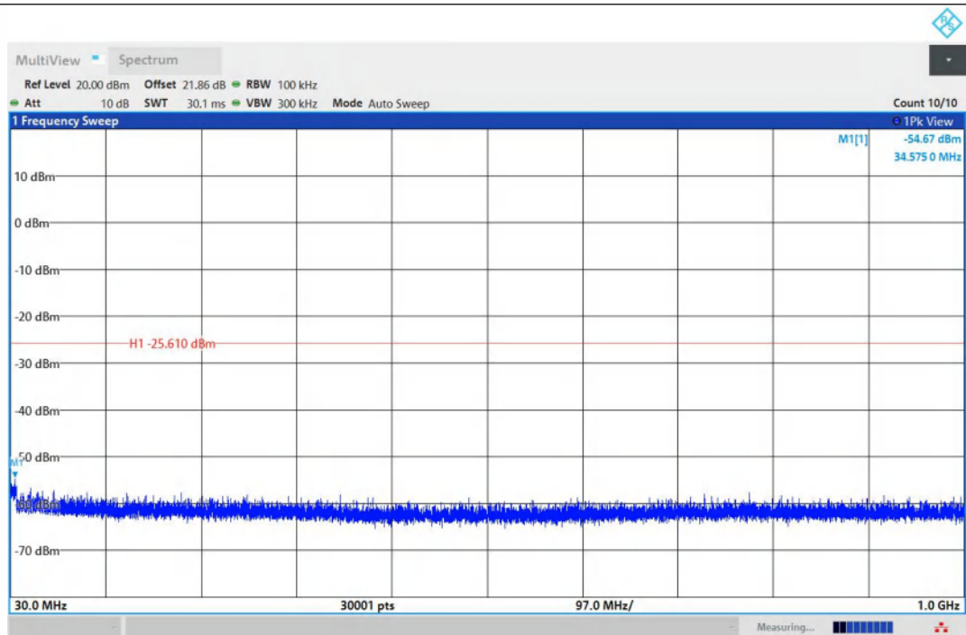
11G-Ant1-2437-30~1000-PASS
