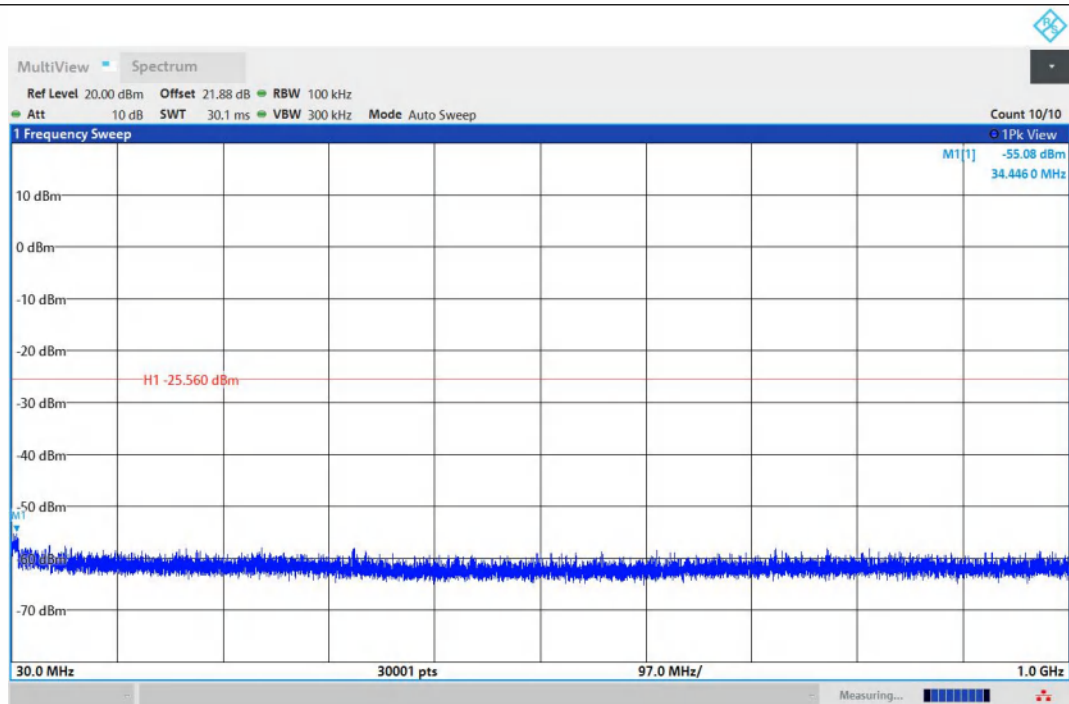
11G-Ant1-2462-30~1000-PASS
