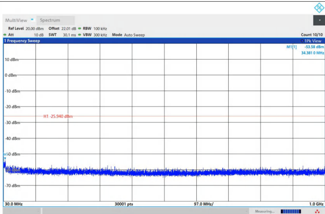
11G-Ant1-2412-30~1000-PASS
