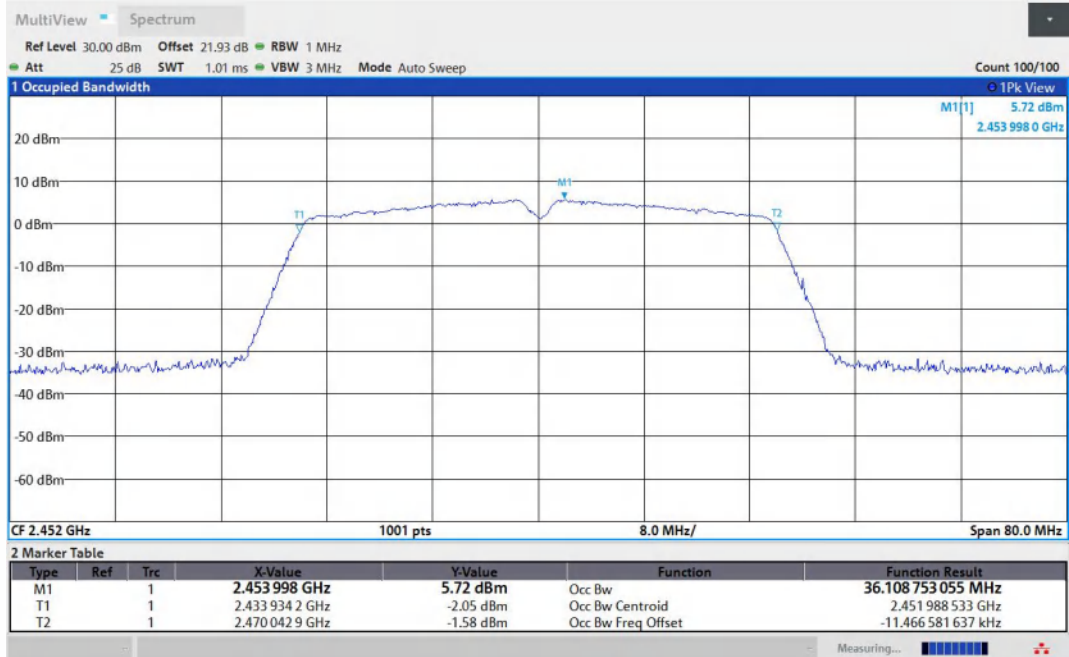
11N40MIMO-Ant1-2452
