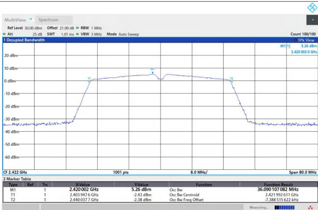
11N40MIMO-Ant1-2422
