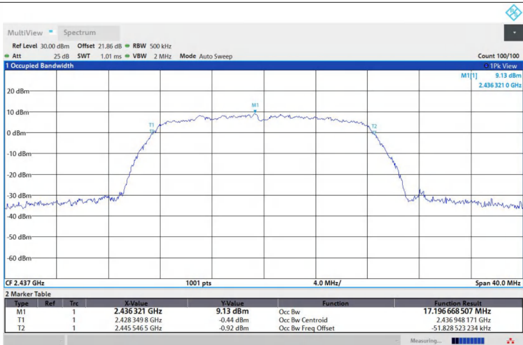
11G-Ant1-2437
