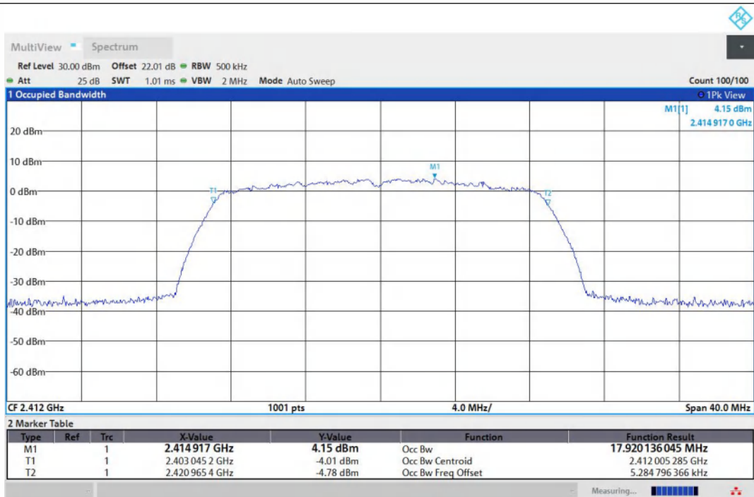
11N20MIMO-Ant1-2412
