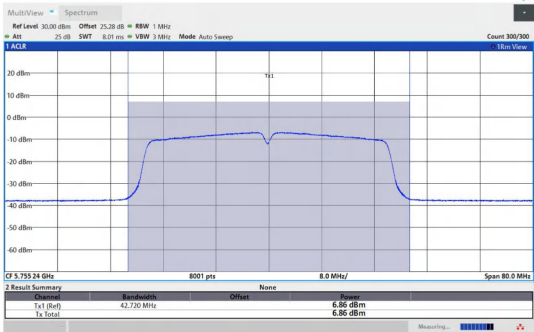
11N40MIMO-Ant1-5755-PASS
