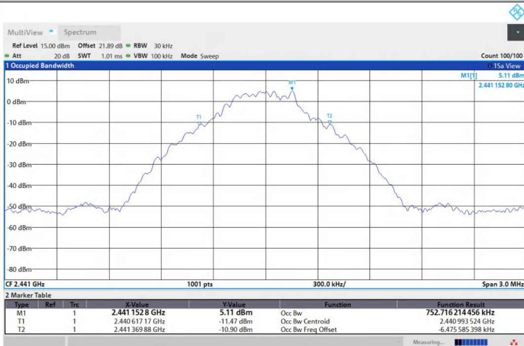
DH5-Ant1-2441
