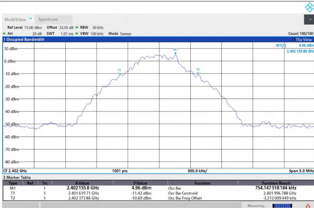
DH5-Ant1-2402
