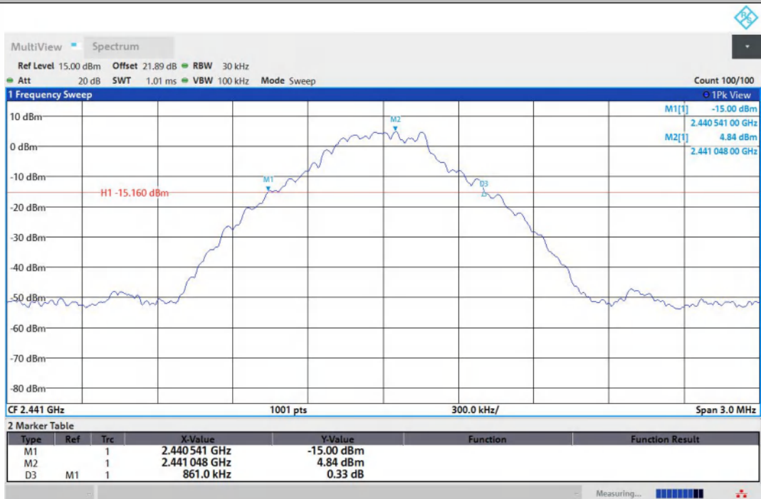
DH5-Ant1-2441
