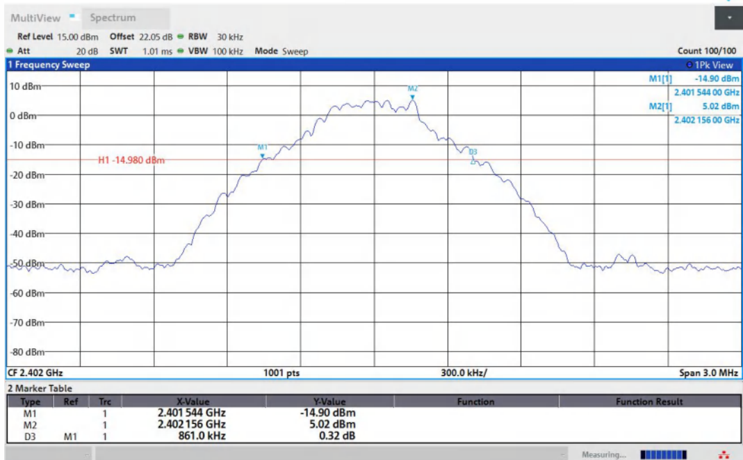
DH5-Ant1-2402
