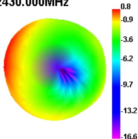
2430.000MHz
