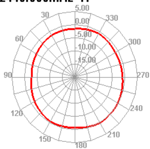
2440.000MHz H
