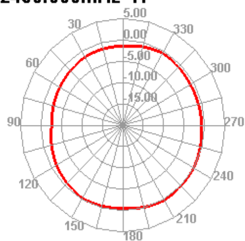
2450.000MHz H
