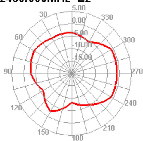
2430.000MHz E2
