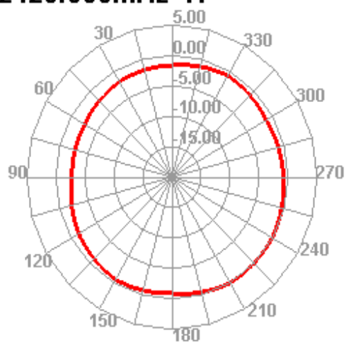
2420.000MHz H
