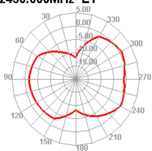
2430.000MHz E1
