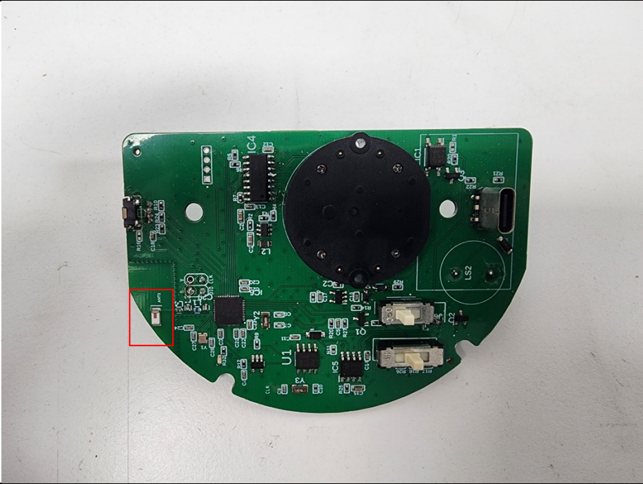
ANTENNA(2.4 GHz)
