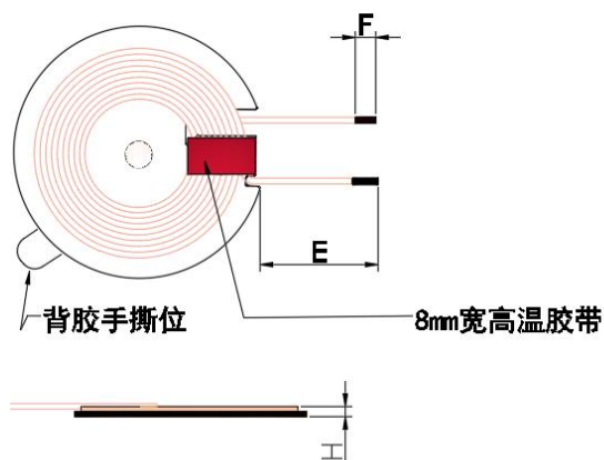
图三、线圈与磁片组合
