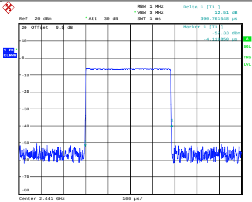
GFSK_Hopping_DH1 0.391ms
