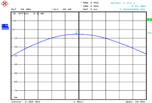
PI/4-DQPSK_Low&-5.61 dBm
