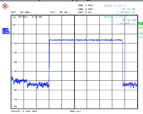
\pi/4 -DQPSK_Hopping_2DH5 2.928ms
