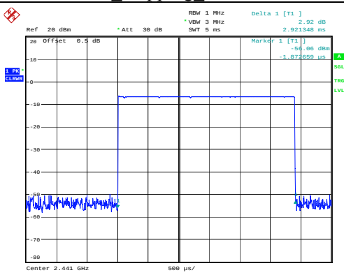
GFSK_Hopping_DH5 2.921ms
