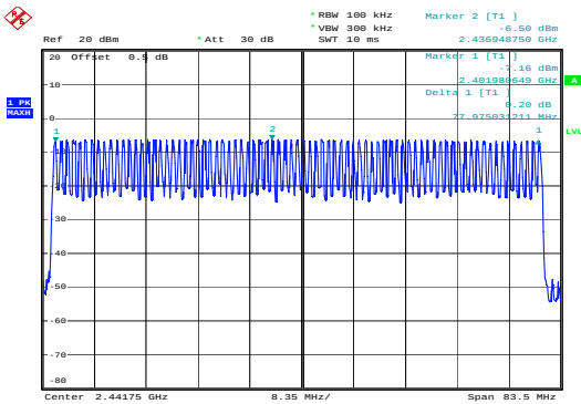
BDR GFSK_Hopping&79
