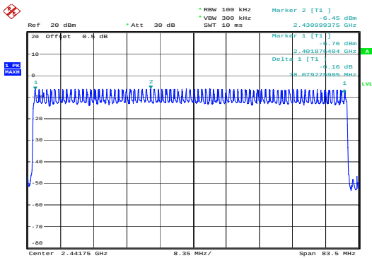
EDR PI/4-DQPSK_Hopping&79
