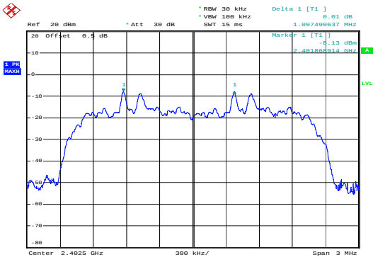
PI/4-DQPSK_Low&1.007 MHz
