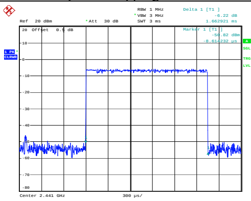
\pi/4 -DQPSK_Hopping_2DH3 1.663ms
