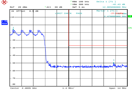
PI/4-DQPSK_Hopping_Upper&42.43 dB
