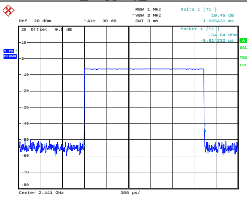
GFSK_Hopping_DH3 1.655ms
