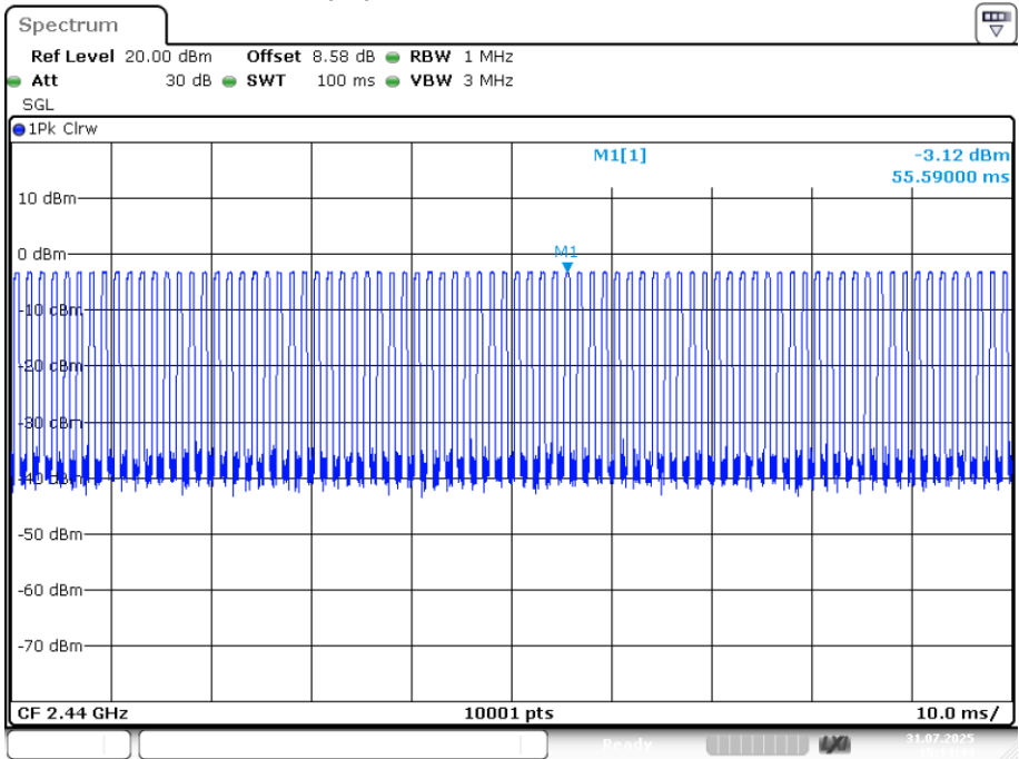
Duty Cycle NVNT BLE 1M 2440MHz Ant1
