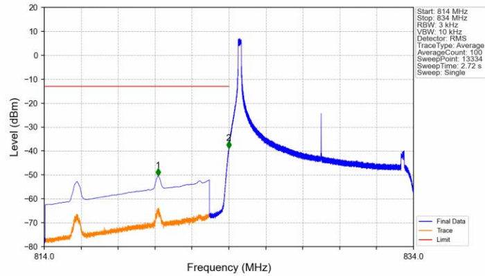
Band5 10MHz QPSK LCH 829MHz RB 1 0 NTNV
