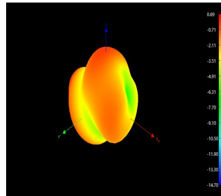
2450MHz 3D
