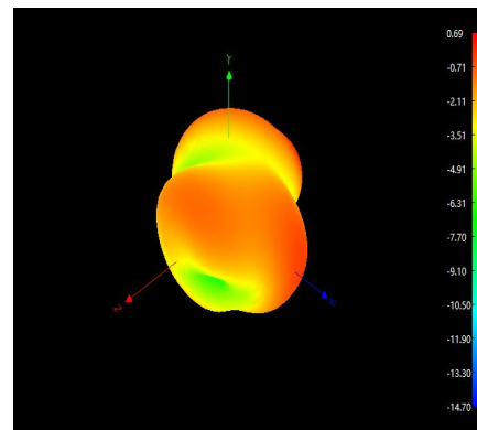
2500MHz 3D
