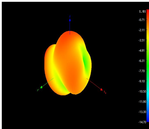
2470MHz 3D
