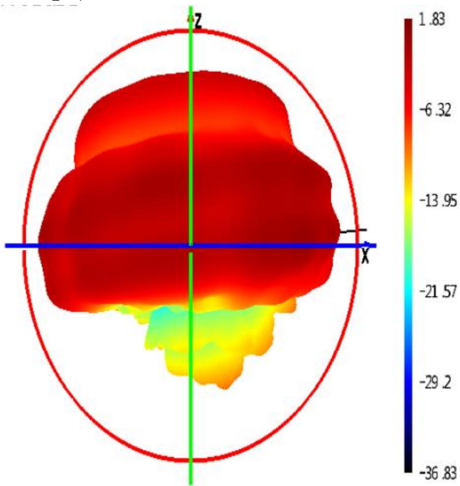
2435MHz 3D_Graphs
