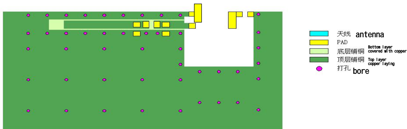
打孔参考示意图 Punching reference diagram
