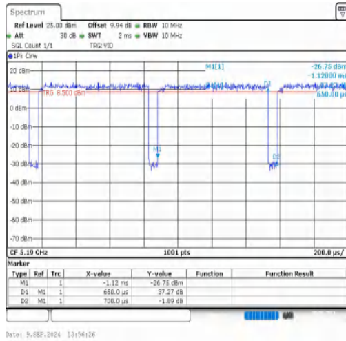
NTNV-11N40MIMO-Ant1-5190
