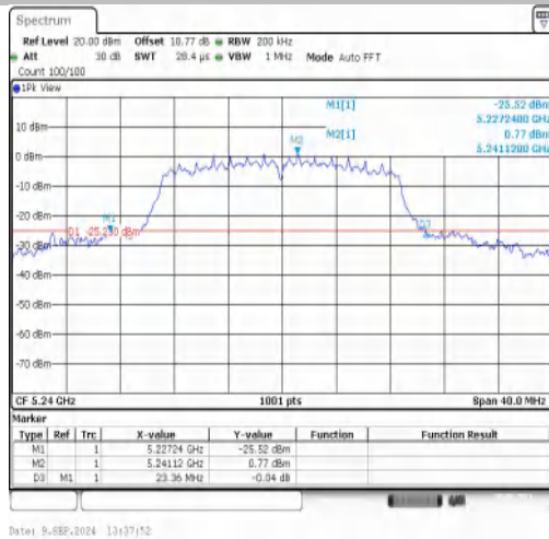
11N20MIMO-Ant1-5240
