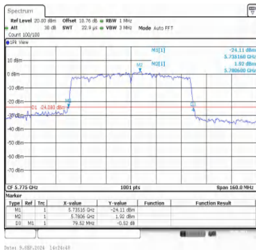
11AC80MIMO-Ant1-5775
