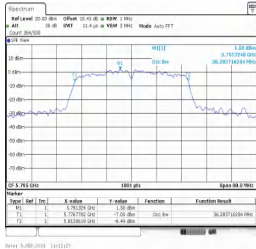
11N40MIMO-Ant2-5795
