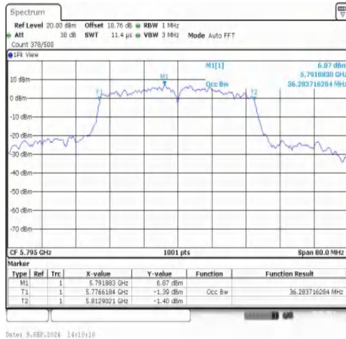
11N40MIMO-Ant1-5795
