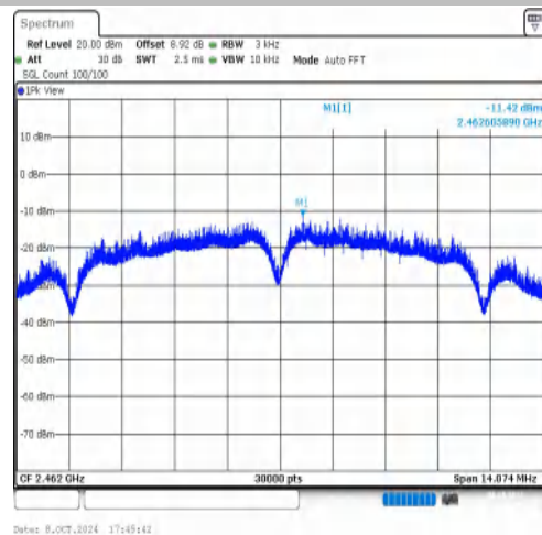
11B-CDD-Ant2-2462-PASS
