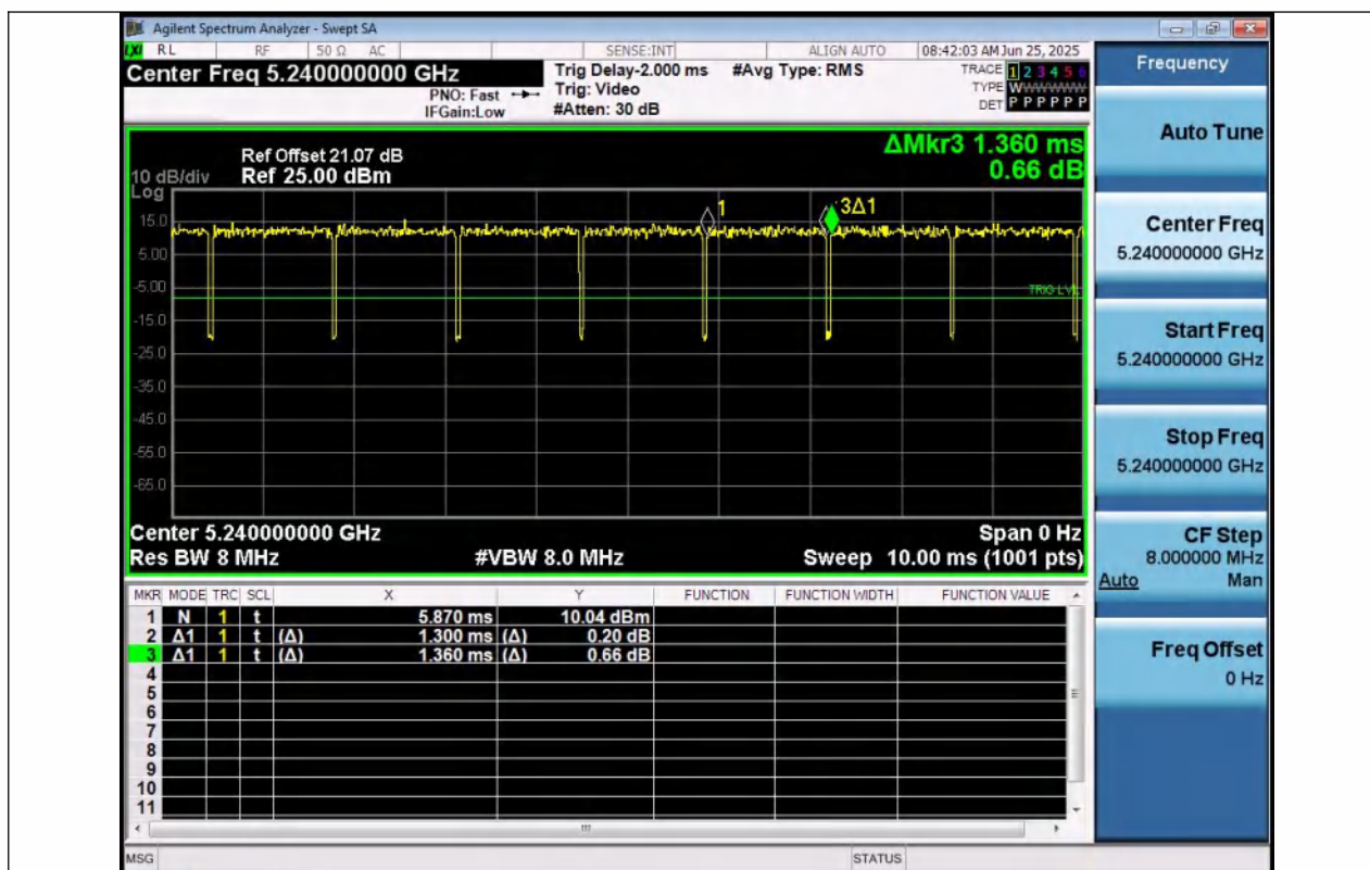
NTNV-11N20MIMO-Ant1-5240
