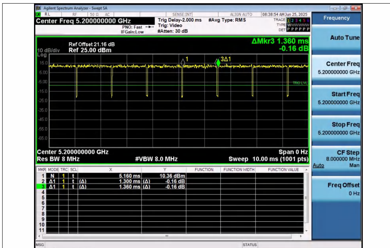
NTNV-11N20MIMO-Ant1-5200
