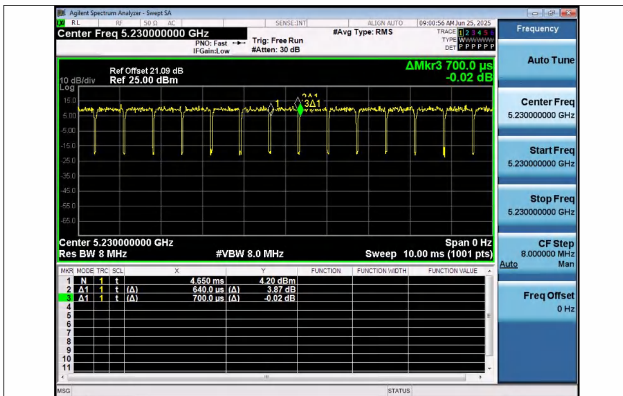
NTNV-11N40MIMO-Ant1-5230
