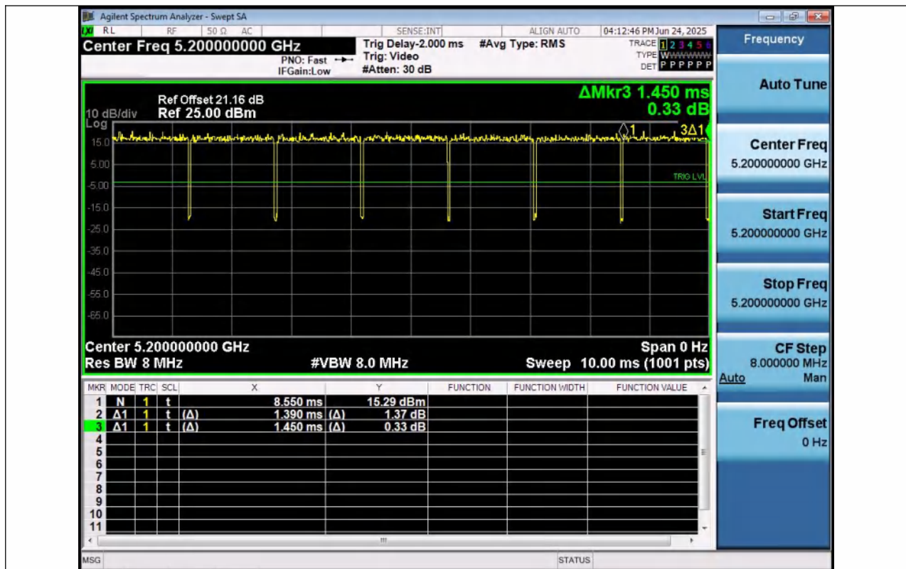
NTNV-11A-Ant1-5200
