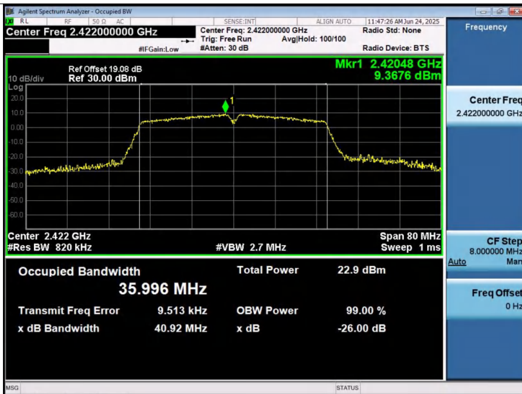
11N40MIMO-Ant1-2422
