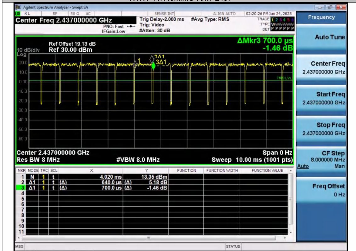
NTNV-11N40MIMO-Ant2-2437
