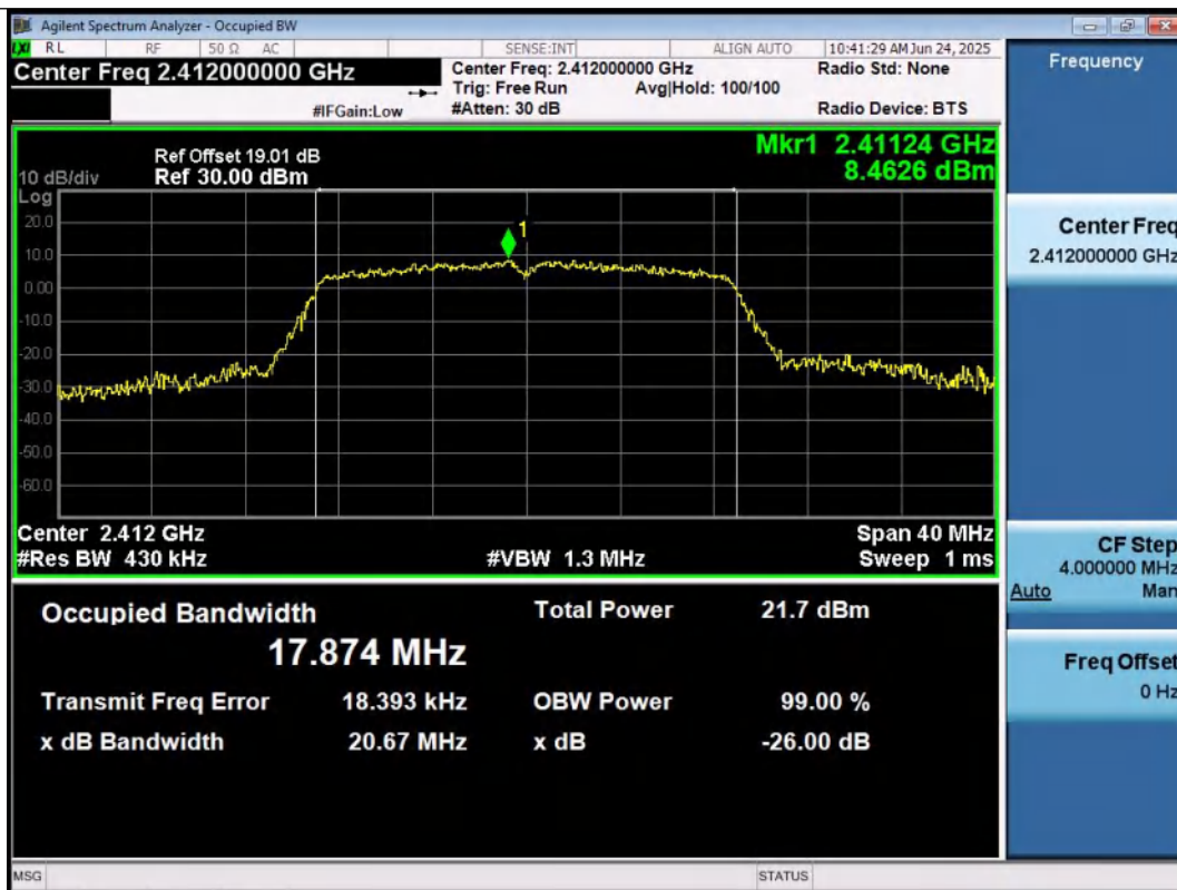
11N20MIMO-Ant1-2412
