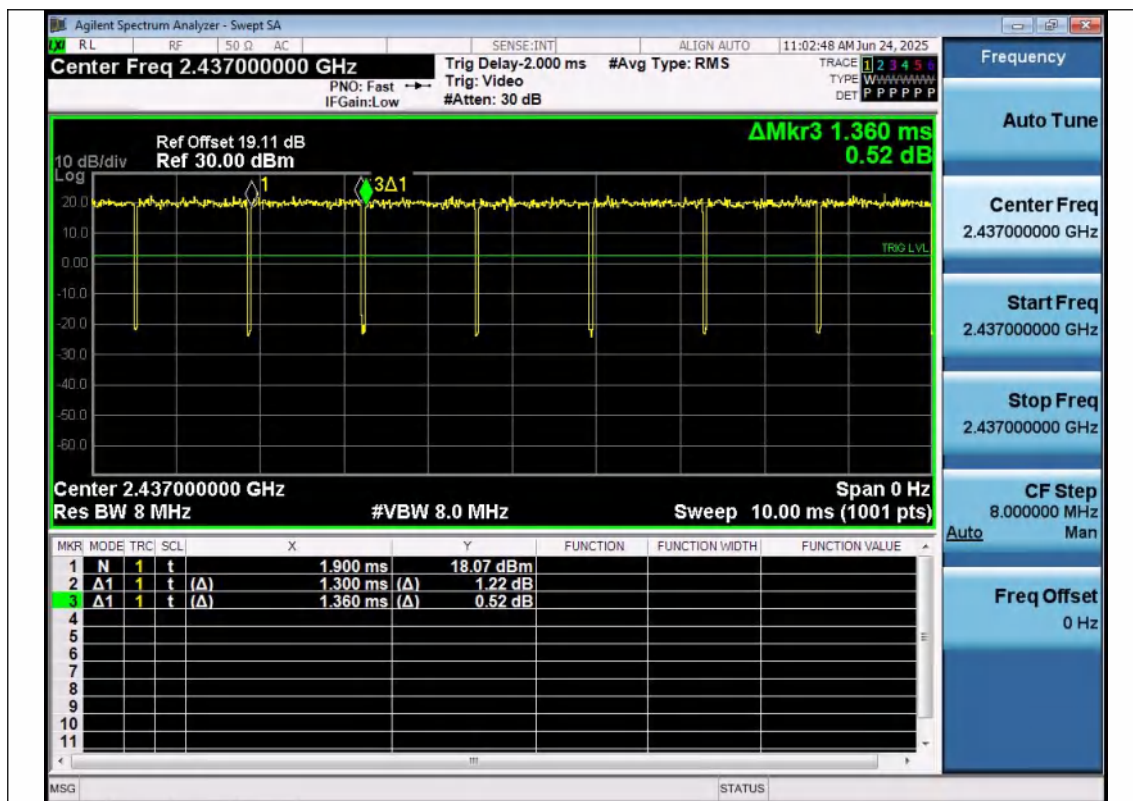
NTNV-11N20MIMO-Ant1-2437
