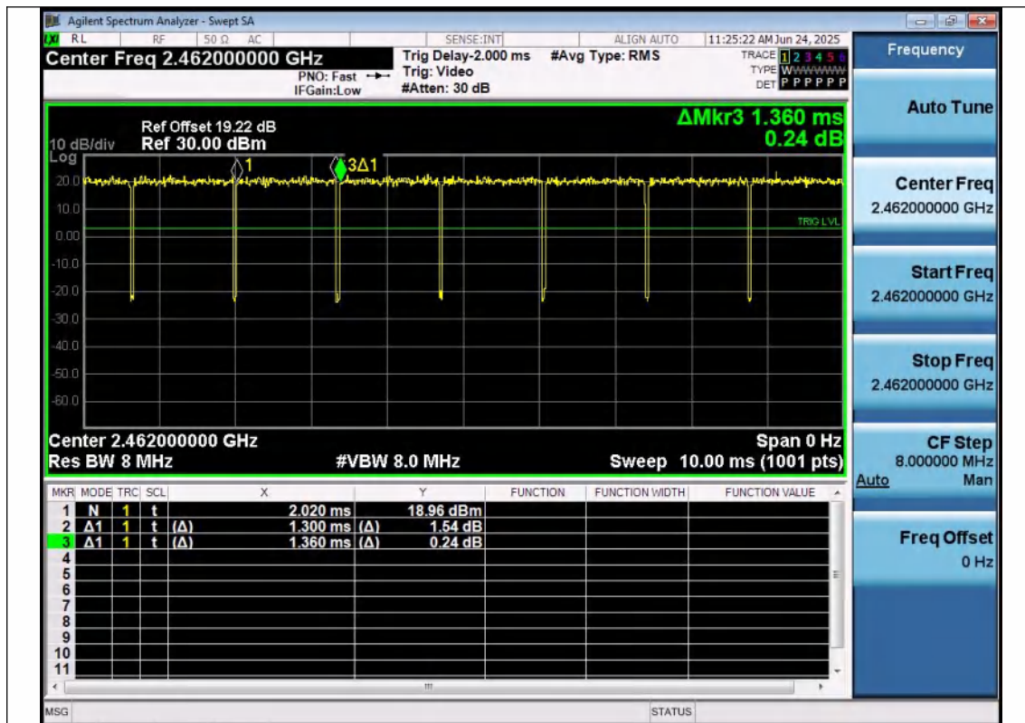
NTNV-11N20MIMO-Ant1-2462
