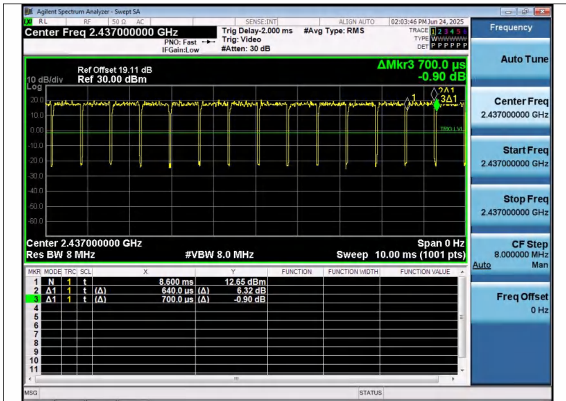
NTNV-11N40MIMO-Ant1-2437
