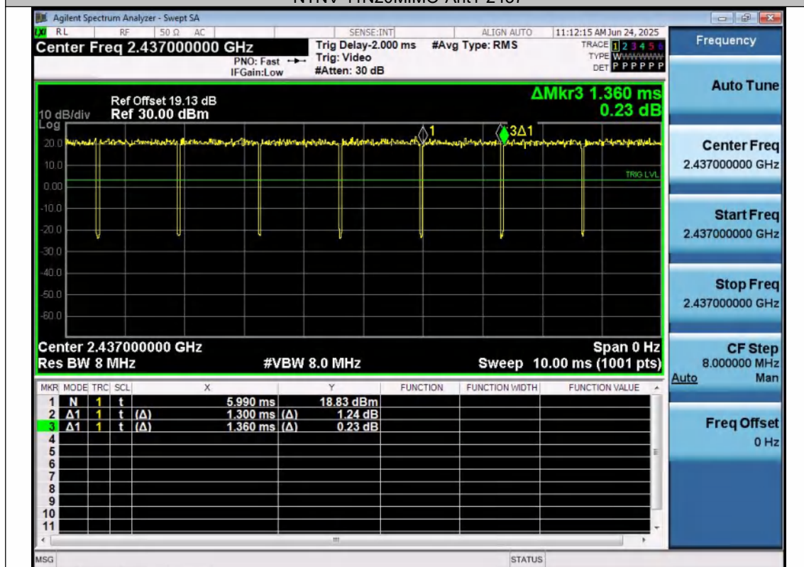
NTNV-11N20MIMO-Ant2-2437
