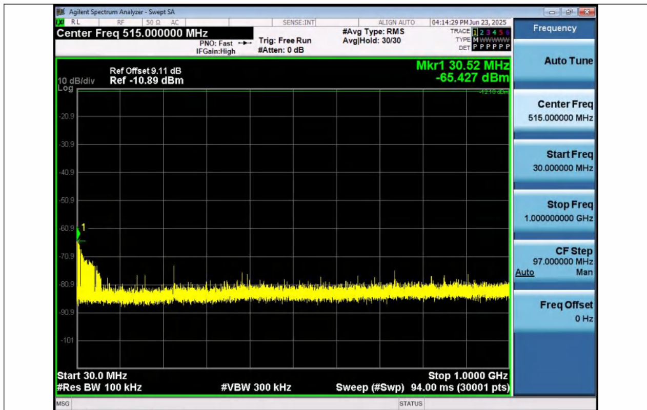
BLE_2M-Ant1-2440-30~1000-PASS
