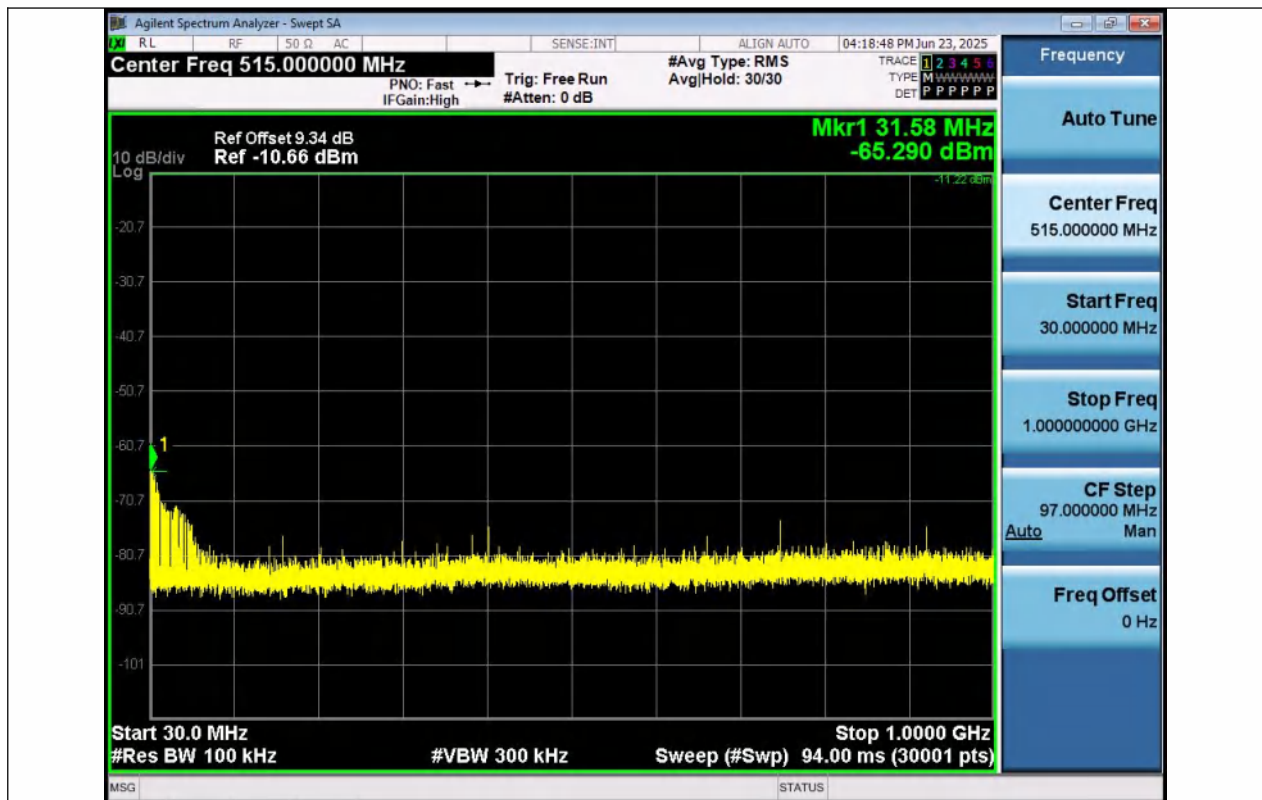
BLE_2M-Ant1-2480-30~1000-PASS
