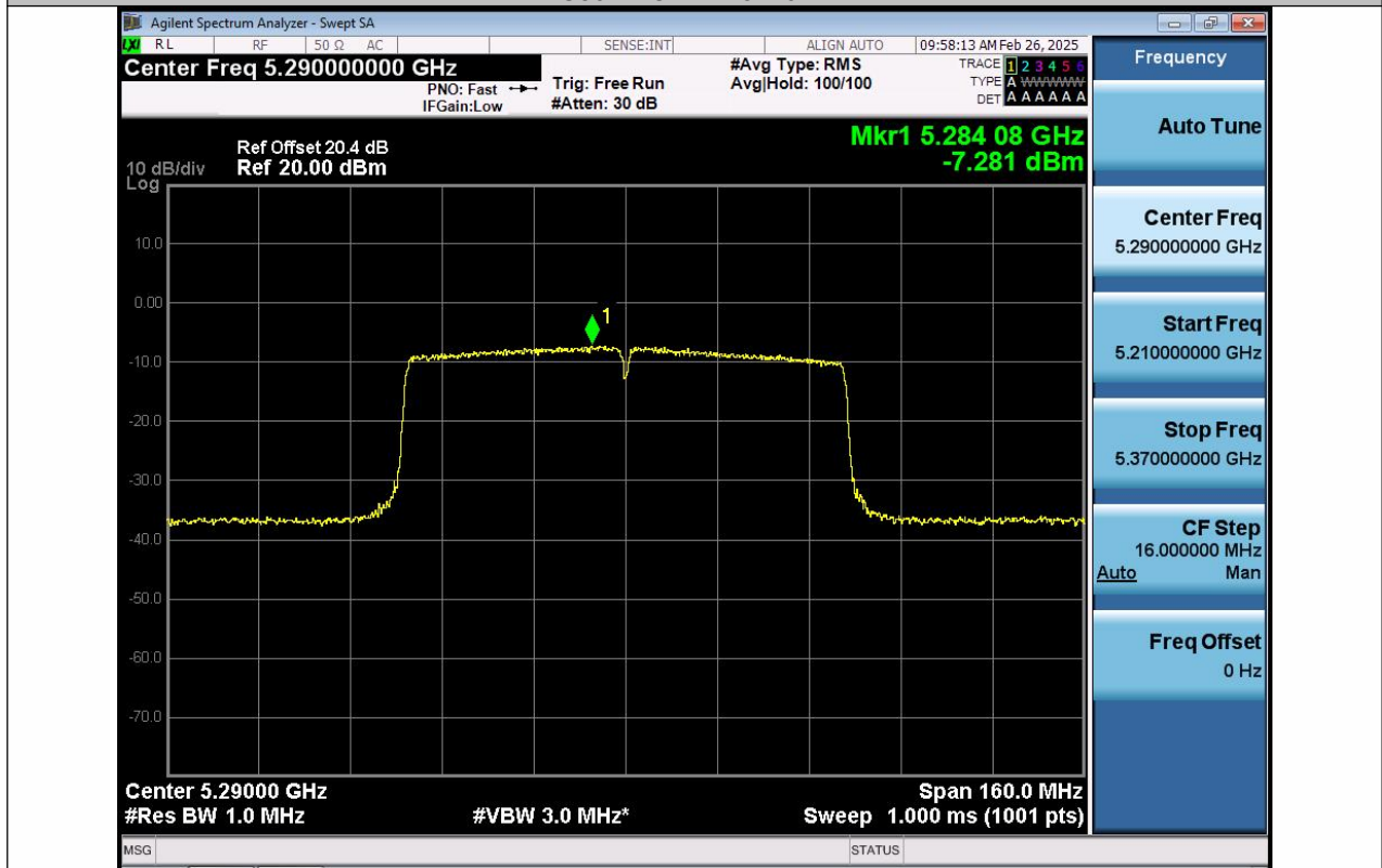
11AC80SISO-Ant1-5290-PASS
