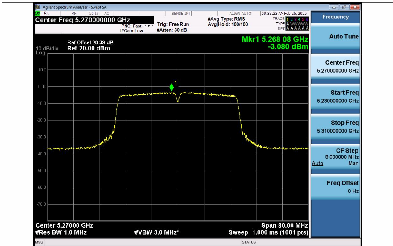
11N40SISO-Ant1-5270-PASS
