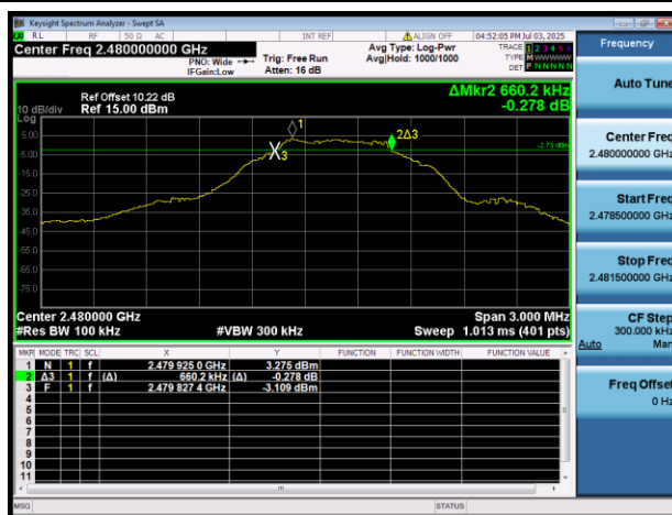
2.4G 2480MHz
