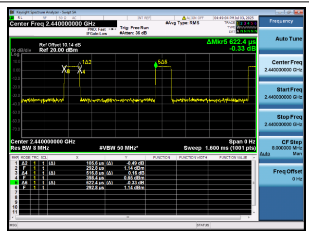
2.4G 2440MHz
