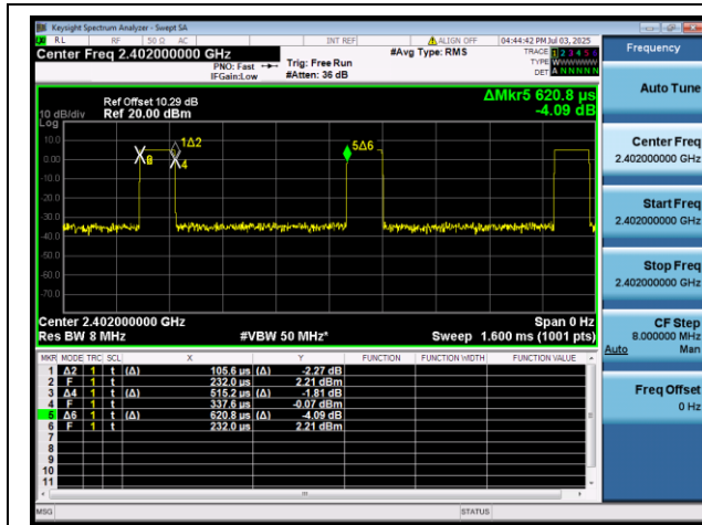
2.4G 2402MHz
