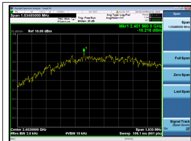
2.4G 2402MHz
