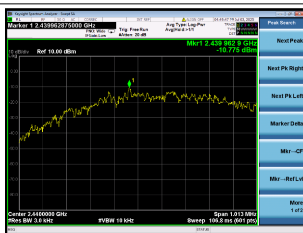
2.4G 2440MHz
