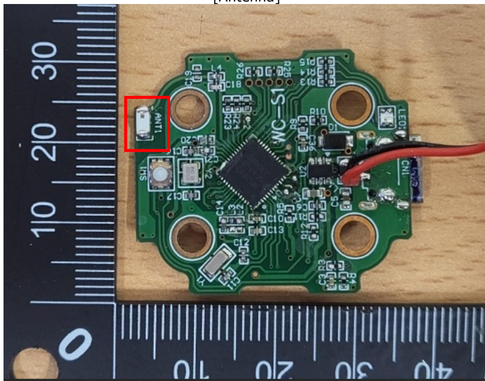
[Antenna]
