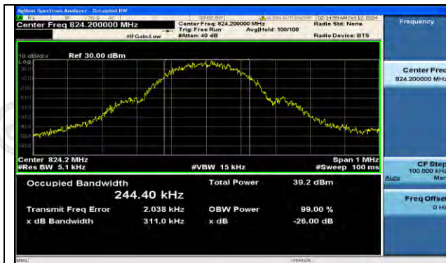
GSM850-128-5-PASS
