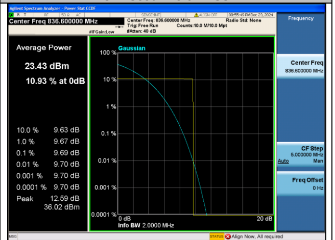
GPRS850-190-5-PASS
