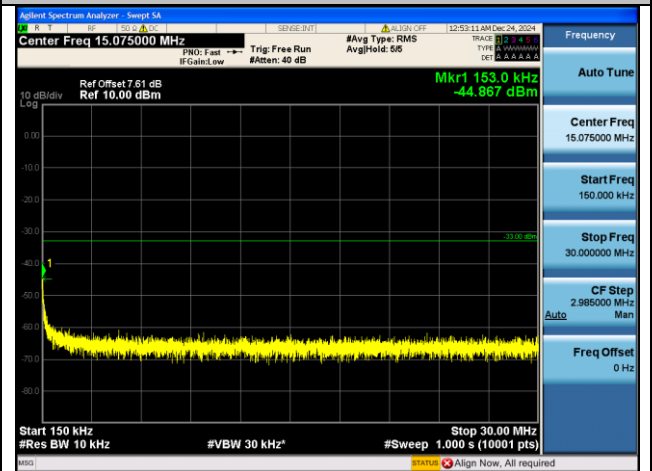
GPRS1900-810-0-0.15-30MHz-PASS
