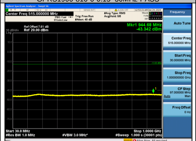
GPRS1900-810-0-30-1000MHz-PASS
