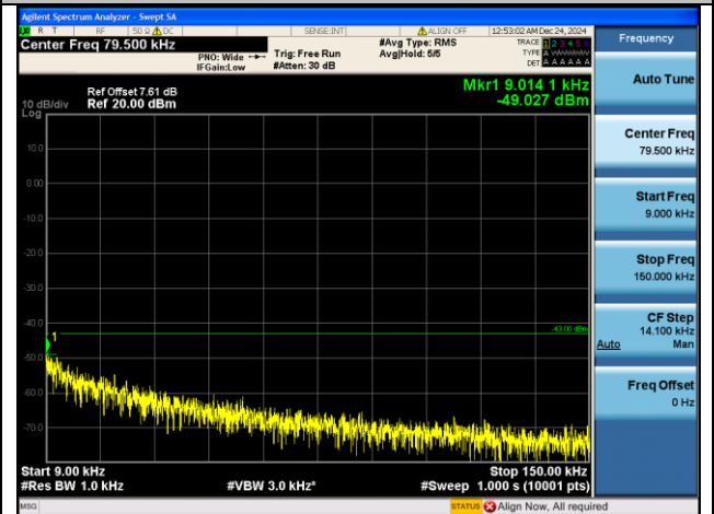
GPRS1900-810-0-0.009-0.15MHz-PASS
