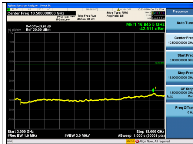
GSM1900-661-0-3000-18000MHz-PASS
