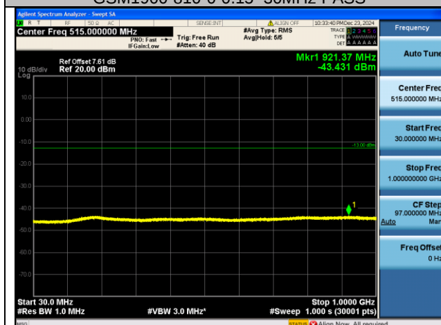
GSM1900-810-0-30-1000MHz-PASS
