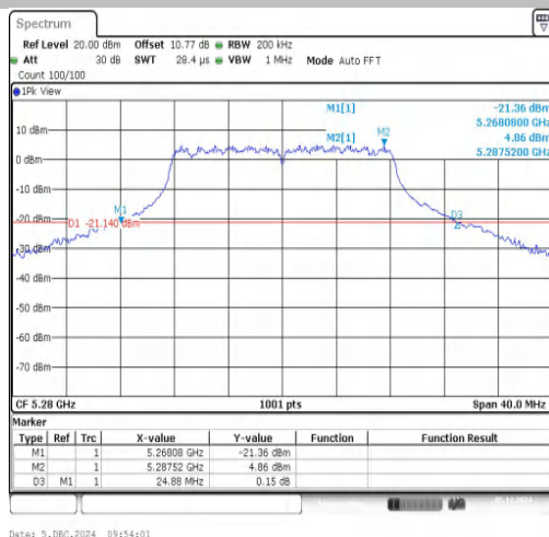
11A-Ant1-5280
