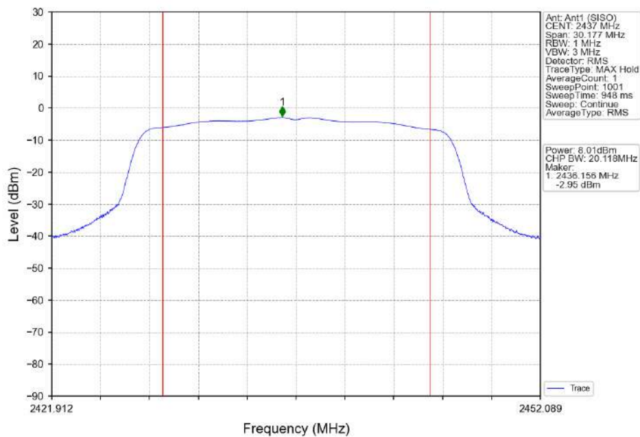
802.11ax(HEW20)_MCH_2437MHz_RU242_Left_Ant1 (SISO) NTNv
