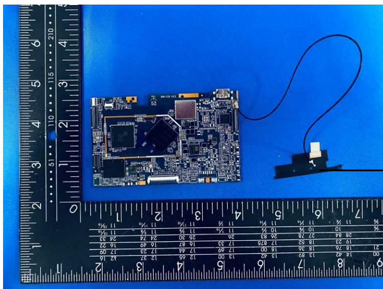
BT/WIFI PIFA Antenna
