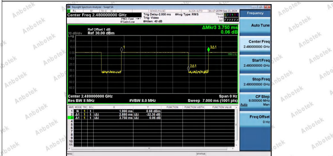
NTNV-DH5-Ant1-2480
