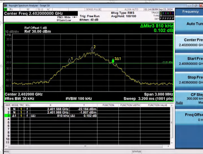
DH5-Ant1-2402
