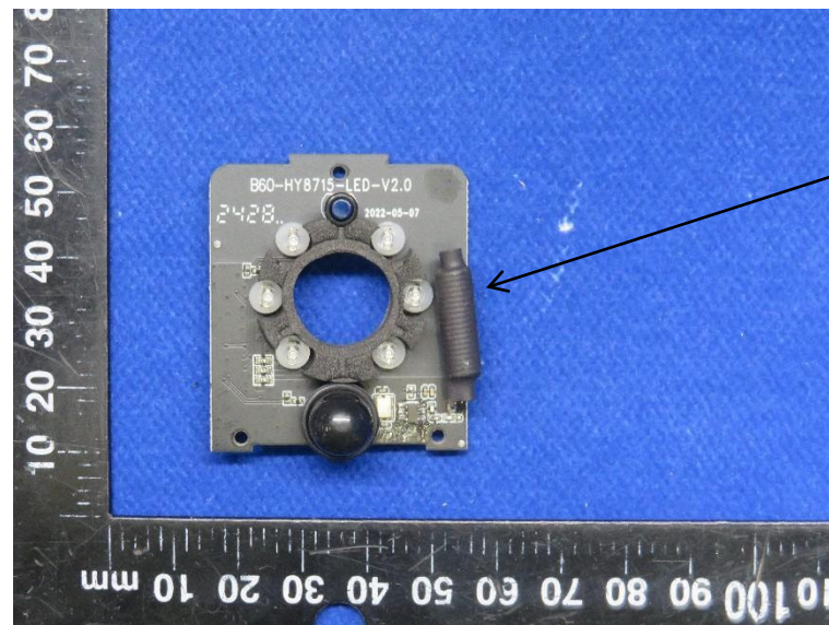
433 TX ANT
