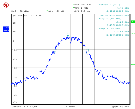
802.11b_2412MHz
