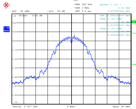
802.11b_2437MHz
