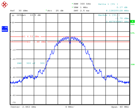
802.11b_2462MHz
