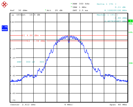
802.11b_2412MHz
