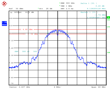
802.11b_2437MHz
