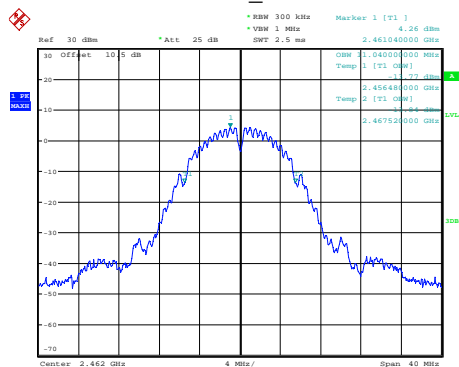
802.11b 2462MHz
