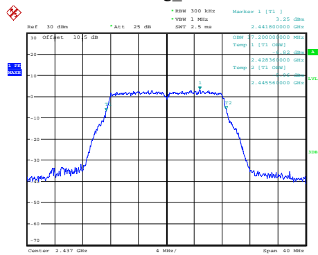
802.11g_2437MHz
