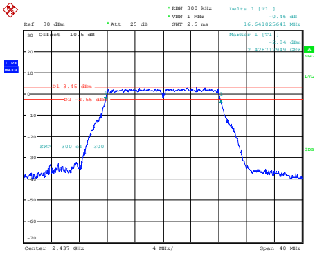
802.11g_2437MHz
