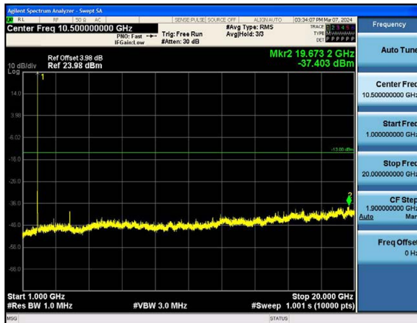
Band2-10MHz-QPSK-18650-1RB#0-Range2:1000~20000MHz
