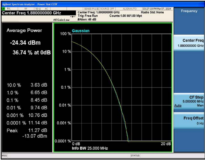
Band2-20MHz-16QAM-19100-1RB#0
