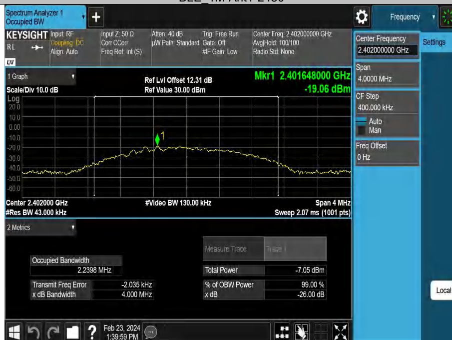
BLE_2M-Ant1-2402
