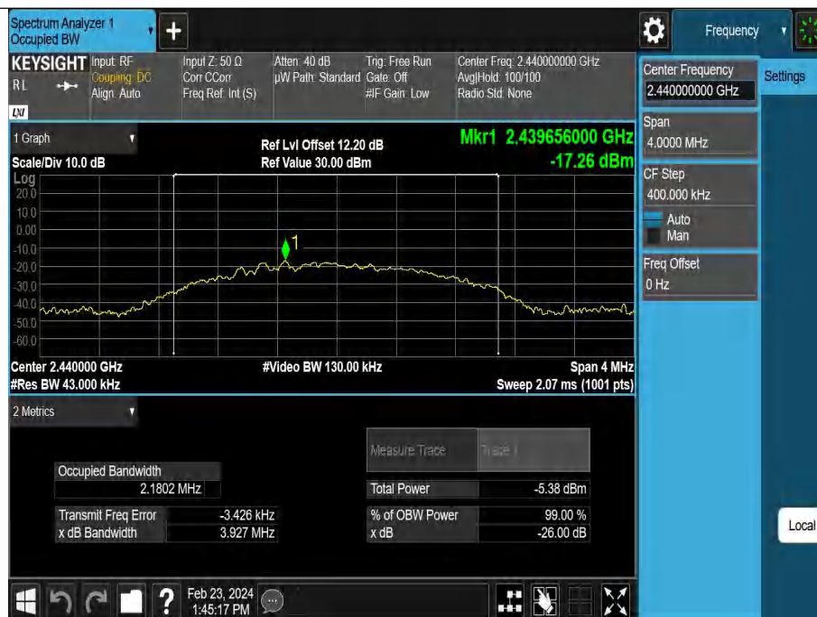
BLE_2M-Ant1-2440
