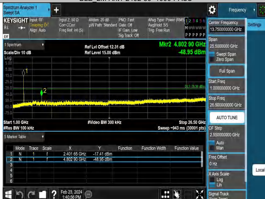
BLE 2M-Ant1-2402-1000~26500-PASS
