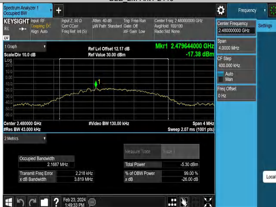
BLE_2M-Ant1-2480
