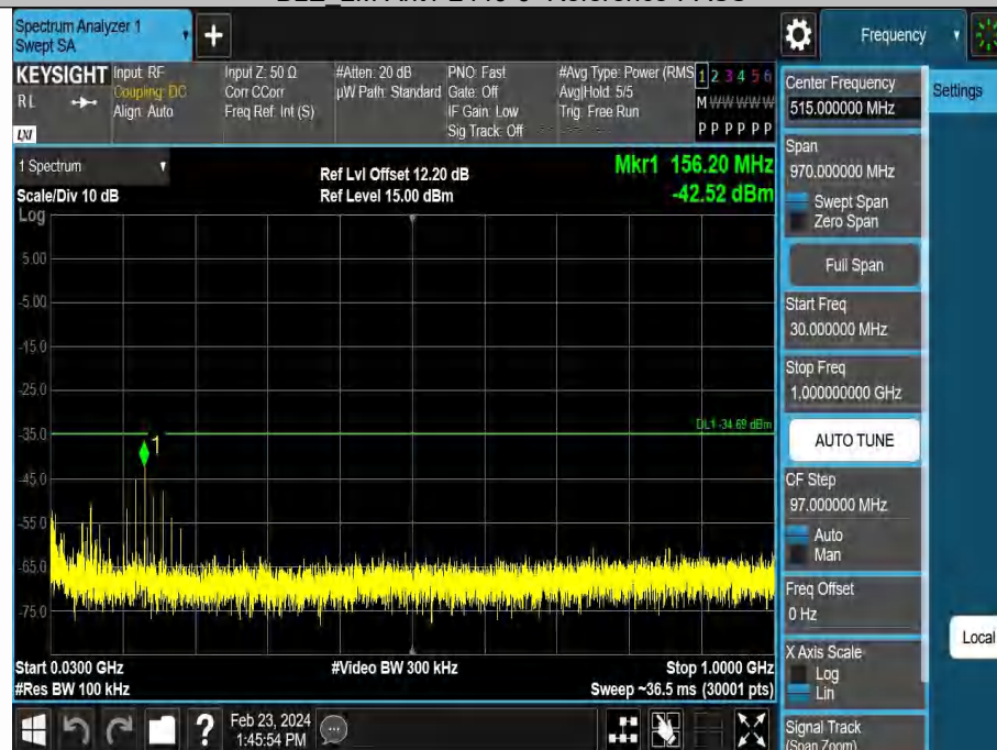
BLE_2M-Ant1-2440-30~1000-PASS
