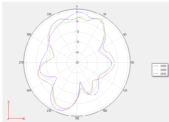
Phi 0 2D图
