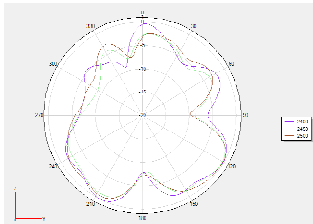
Phi 90 2D图
