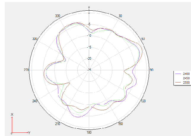
Theta 90 2D图
