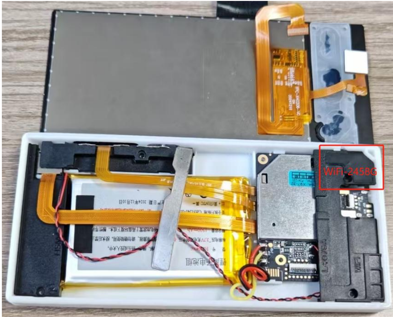
天线安装位置图
