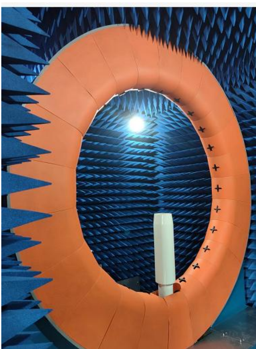
24 探头微波暗室测试设备
