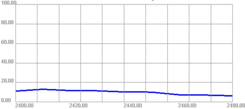
2400.00MHz - 2480.00MHz Efficiency
