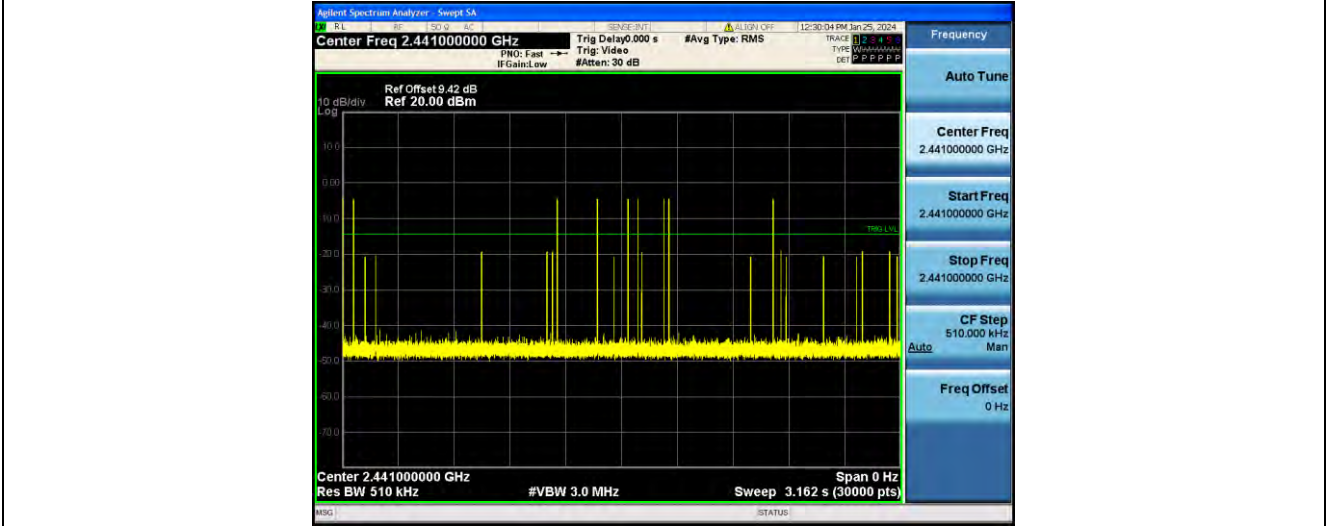
3DH1_Ant1_Hop
