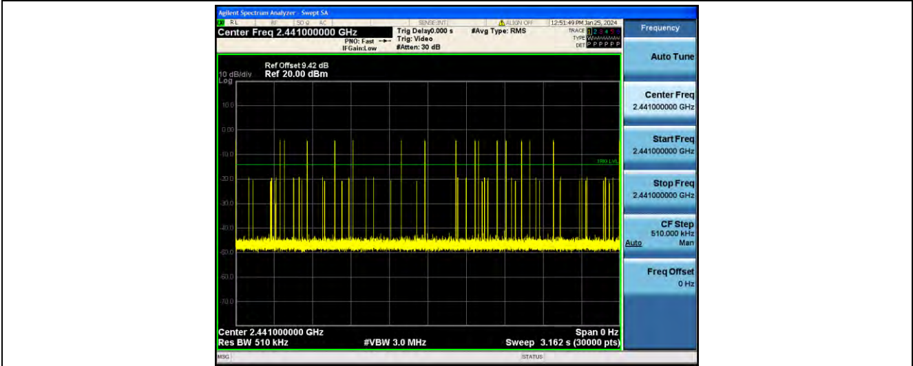
2DH5_Ant1_Hop
