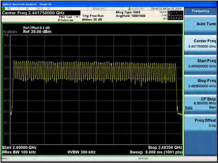
2DH5_Ant1_Hop
