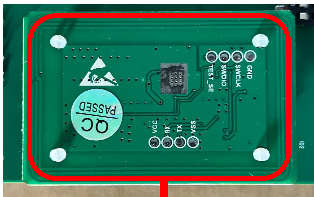
Antenna
