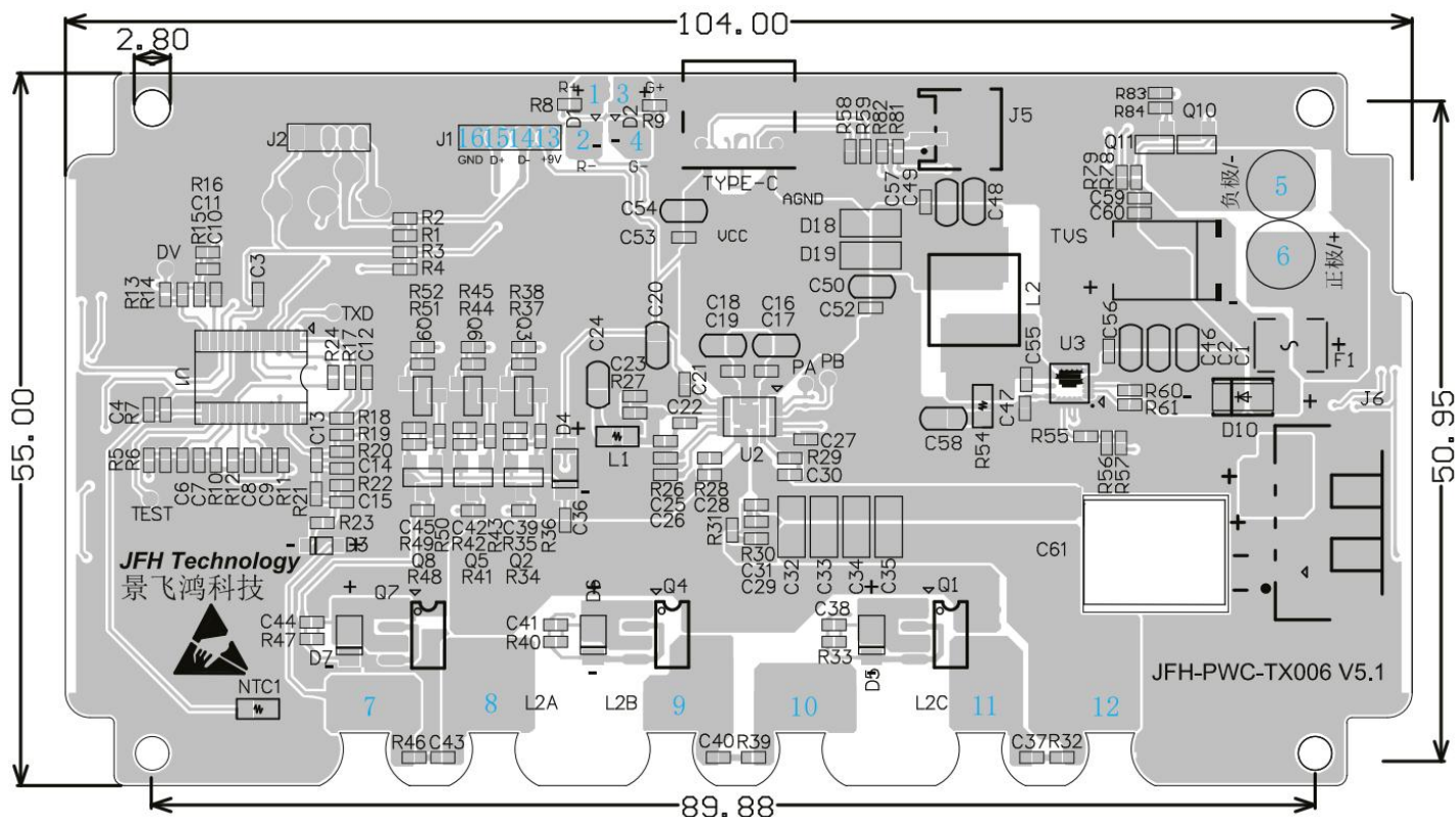
PCB 图
