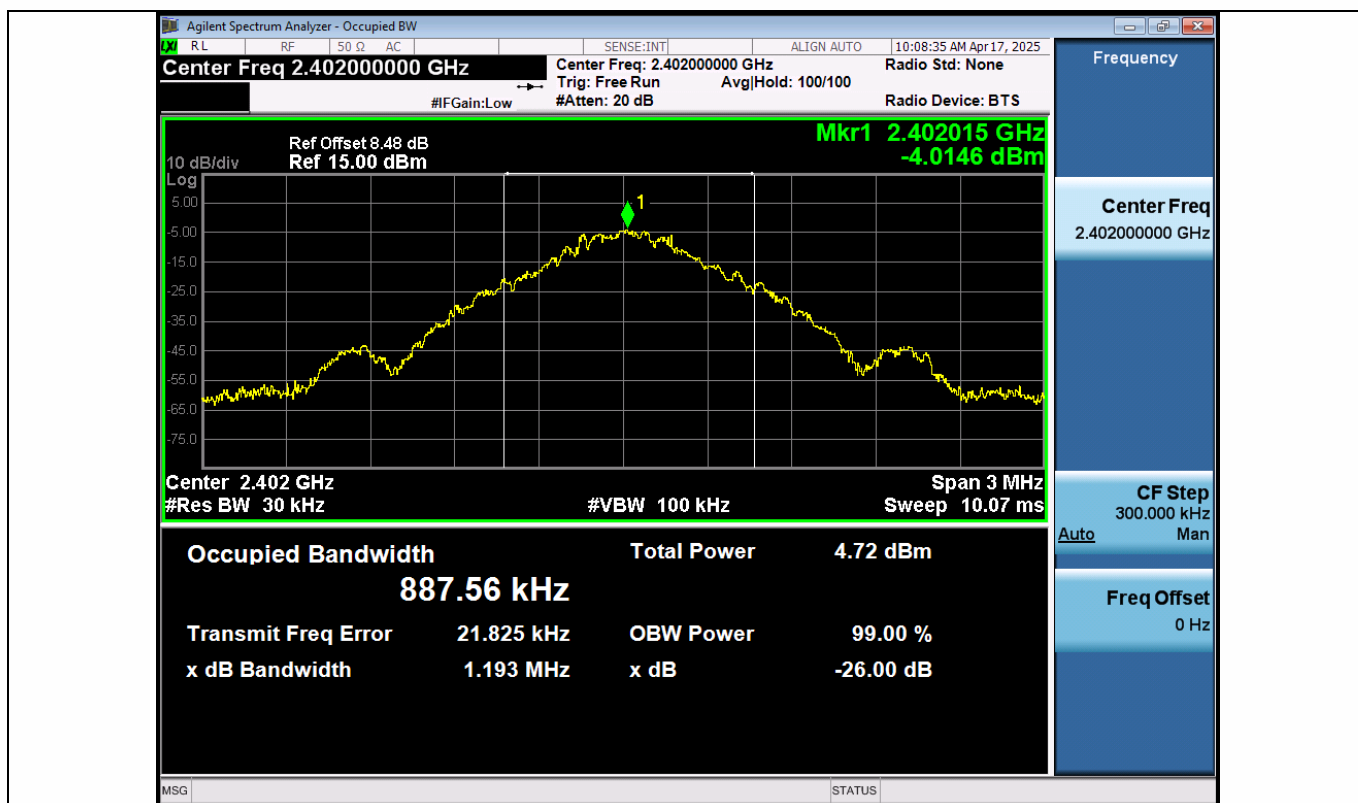
DH5-Ant1-2402
