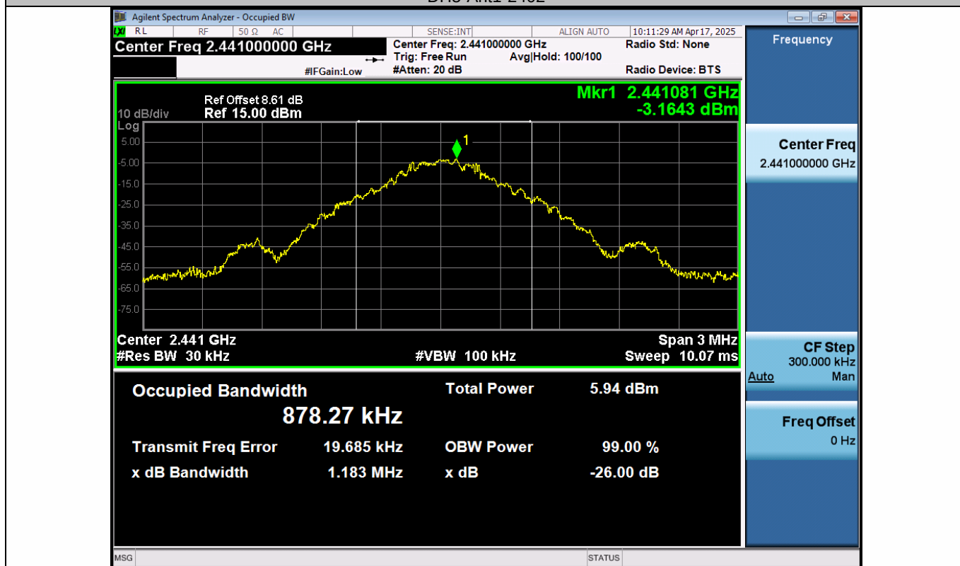
DH5-Ant1-2441
