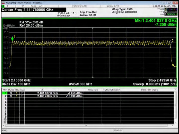
\pi/4 -DQPSK
