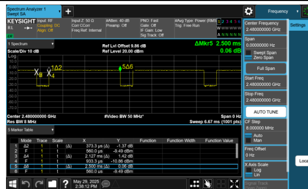
BLE 1Mbps 2480MHz
