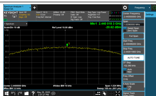
BLE 1Mbps 2440MHz
