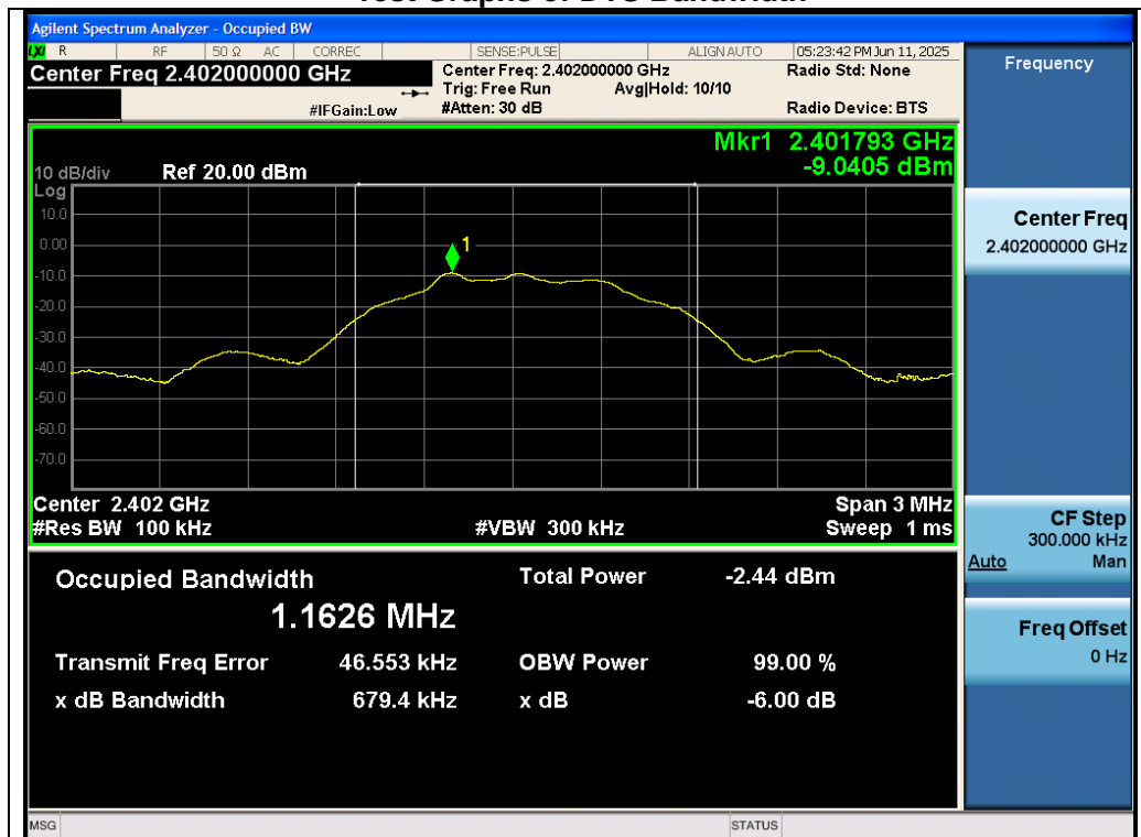
Test_Graph_SRD_ANT1_2402_DTBSW
