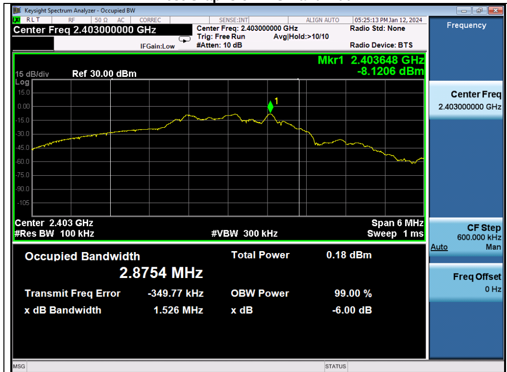
Test_Graph_GFSK_ANT1_2403_2Mbps_DTSBW
