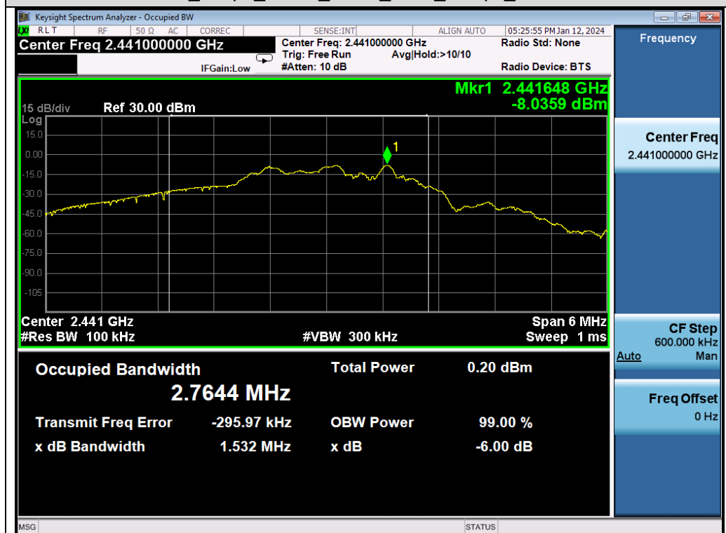
Test_Graph_GFSK_ANT1_2441_2Mbps_DTSBW
