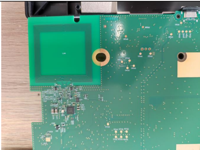
NFC antenna
