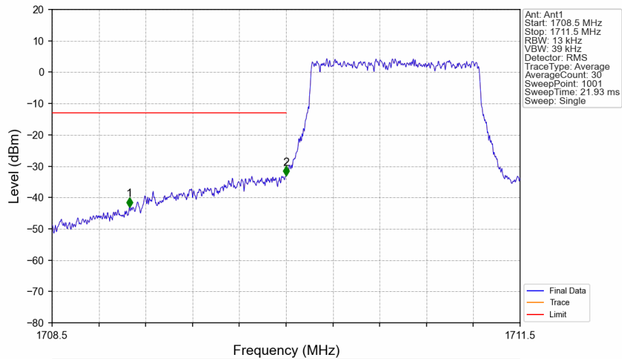
Band4 1.4MHz 16QAM LCH 1710.7MHz RB 6 0 NTV
