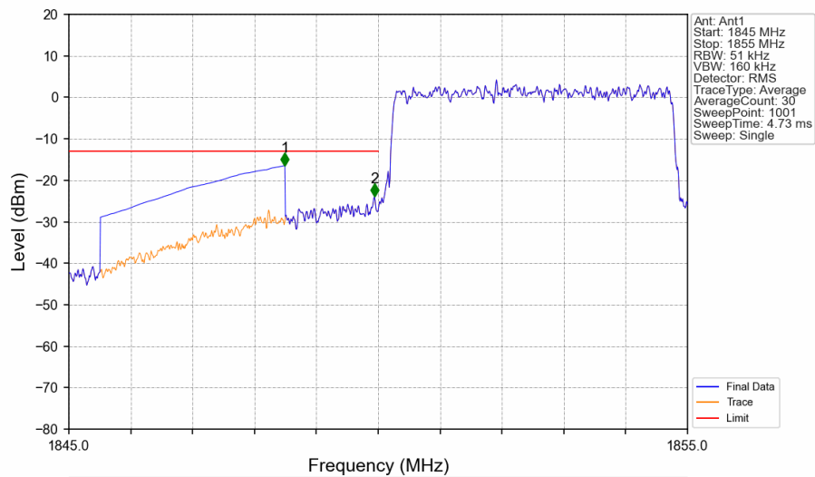
Band2 5MHz 16QAM LCH 1852.5MHz RB 25 0 NTV
