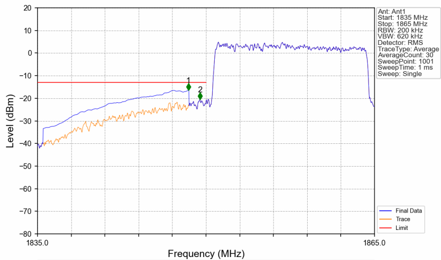
Band2 15MHz 16QAM LCH 1857.5MHz RB 75 0 NTNV
