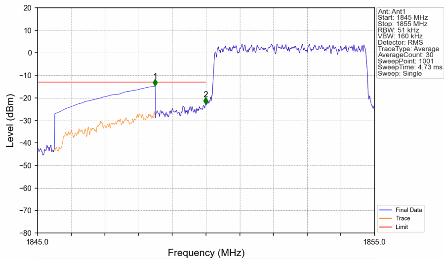
Band2 5MHz QPSK LCH 1852.5MHz RB 25 0 NTN
