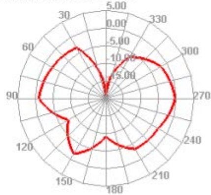
5850.000MHz H
