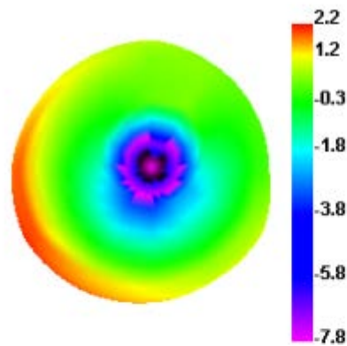
5850.000MHz E1
