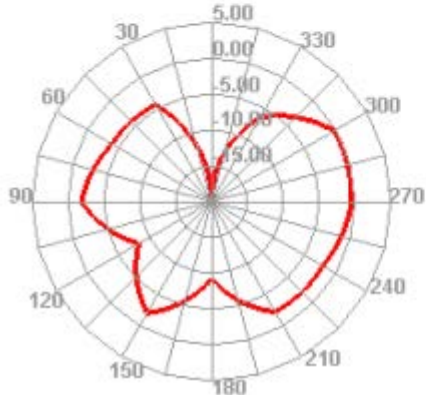
5850.000MHz
